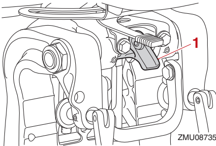
1. Kippsperrhebel
