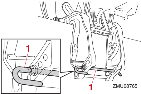
1. Trimmstange
