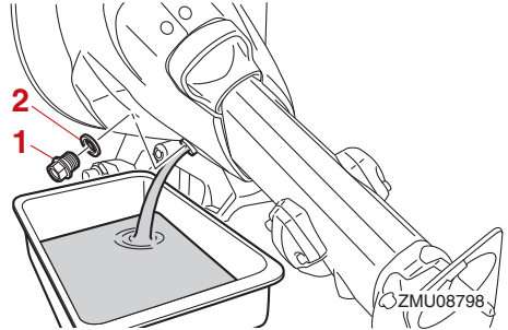
1. Ablassschraube 2. Dichtung
