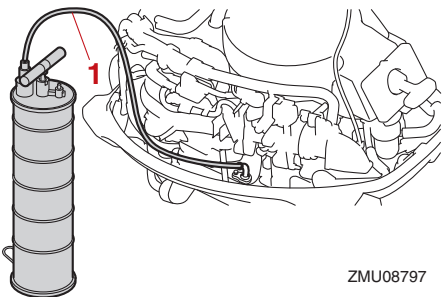
1. Ölwechsler
