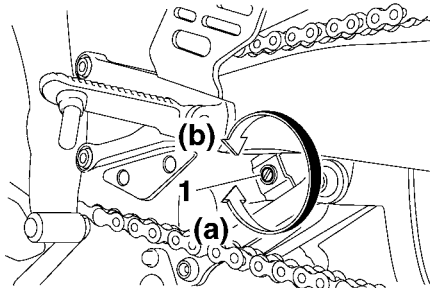
1. Zugstufendämpfungs-Einstellschraube
