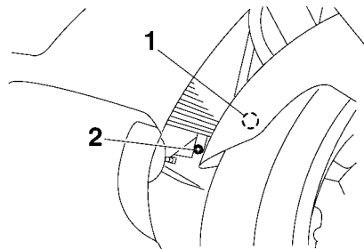
1. Schnellverschluss 2. Schnellverschlusssschraube
