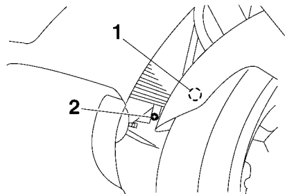
1. Schnellverschluss 2. Schnellverschlusssschraube
