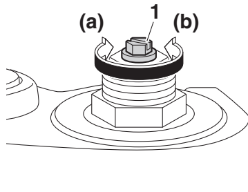
1. Zugstufendämpfungs-Einstellschraube
