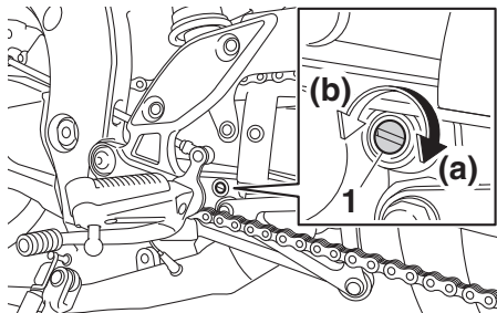
1. Zugstufendämpfungs-Einstellschraube
