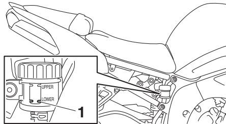
1. Minimalstand-Markierung
