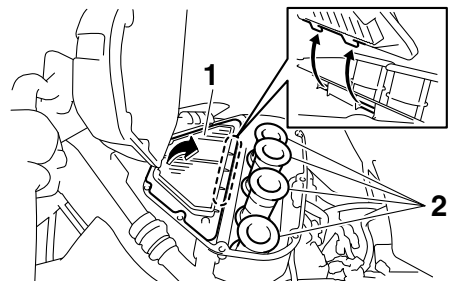
1. Luftfiltereinsatz 2. Einlasskrümmer
