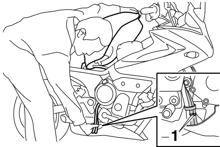
1. Ausgangsstellung (Farbmarkierung)
