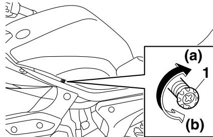
1. Leerlaufeinstellschraube
