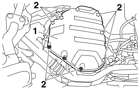
1. Luftfiltergehäuseabdeckung 2. Schraube
