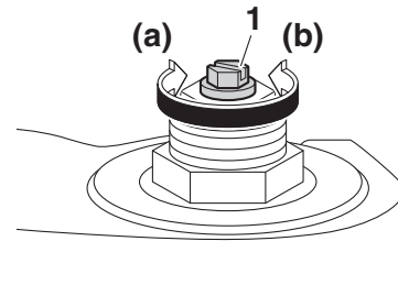
1. Einstellschraube (Zugstufen-Dämpfungskraft)
