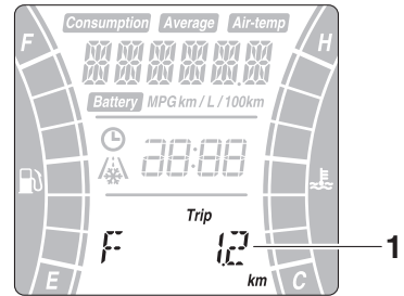
1. Kraftstoffreserve-Kilometerzähler
