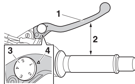
1. Handbremshebel 2. Abstand zwischen Handbremshebel und Gasdrehgriff 3. Einstellrad der Handbremshebelposition 4. Passmarkierung
