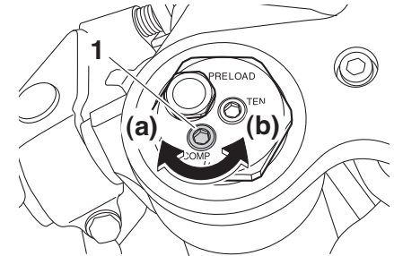
1. Druckstufendämpfungs-Einstellschraube
