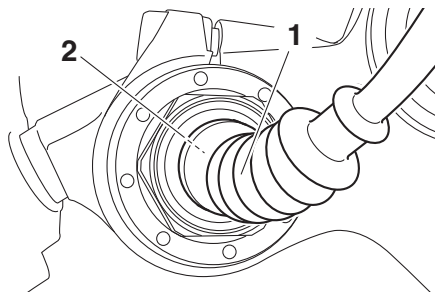
1. Einstellschraube (Federvorspannung)
