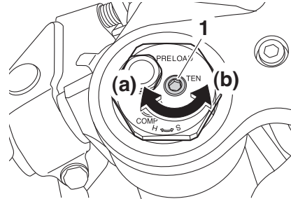
1. Einstellschraube (Zugstufen-Dämpfungskraft)
