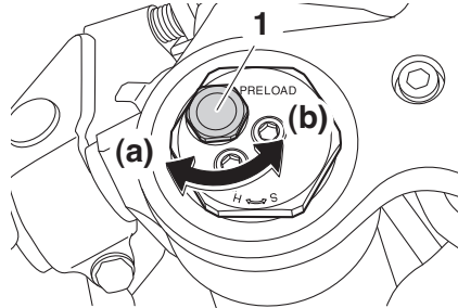
1. Einstellmutter (Federvorspannung)
