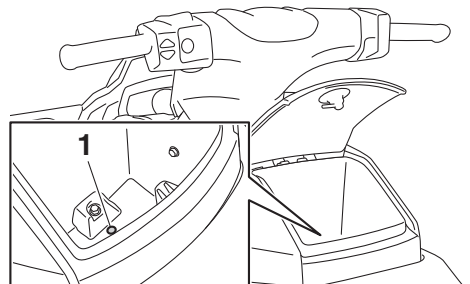
1 Ablassschraube
