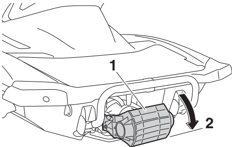
1 Umkehrklappe 2 Rückwärtsstellung
