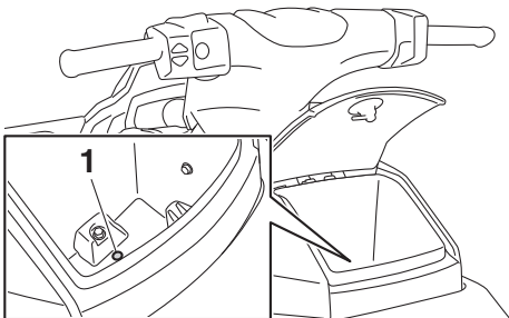
1 Ablassschraube
