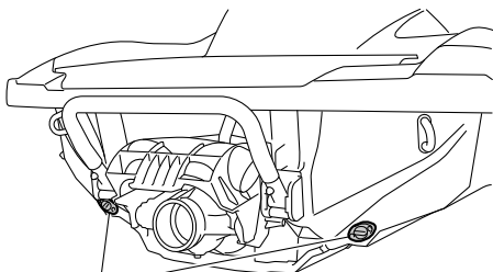
1 Heck-Ablassschraube
