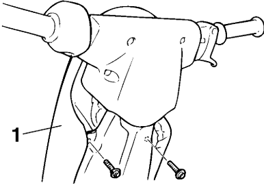
1 Steuermast-Abdeckung
