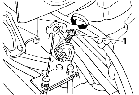
1 Leerlauf-Regulierschraube
