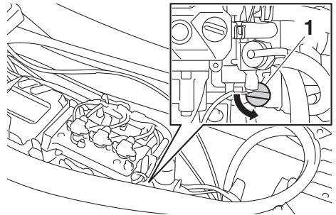
1 Öltankdeckel/Messstab
