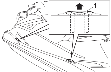
1 Hochklappbare Klampe
