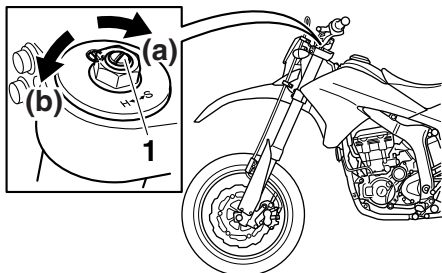
1. Zugstufendämpfungs-Einstellschraube
