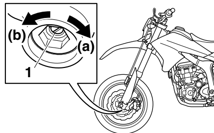
1. Druckstufendämpfungs-Einstellschraube
