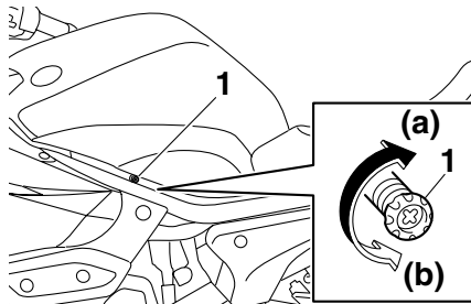
1. Leerlaufeinstellschraube
