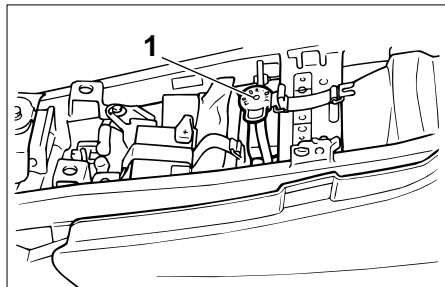
1. Frischöltankverschluß
