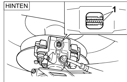
1. Scheibenbremsbelag-Verschleißanzeiger
