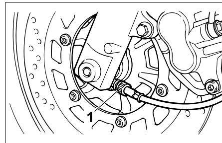
1. Tachowelle
