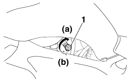
1. Leerlauf­einstellschraube
