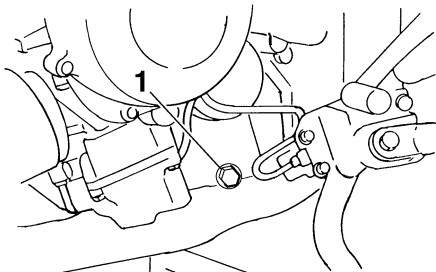
1. Motoröl-Ablasschraube
