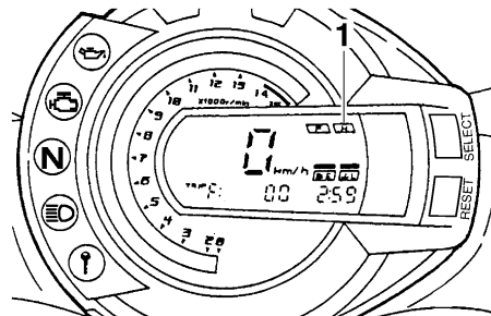
1. Kühflüssigkeitstemperatur-Anzeiger
