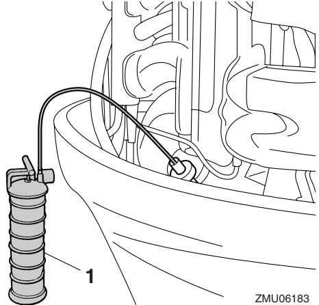
1. Ölwechsler
