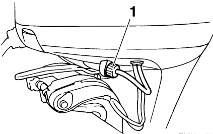
1. Spülanschluss
