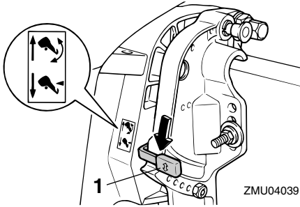
1. Kipperrhebel
