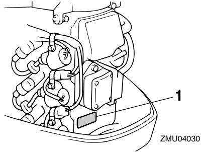
1. Anerkennungsaufkleber-Position
