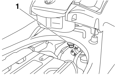
1 Wasserabscheider
