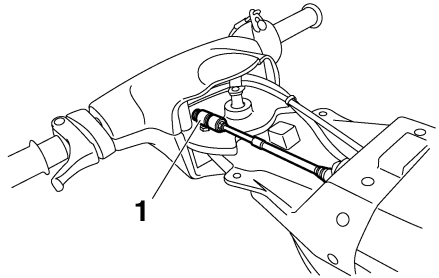
1 Steuerseilzug-Gelenk
