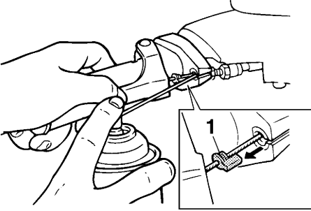
1 Dichtring
