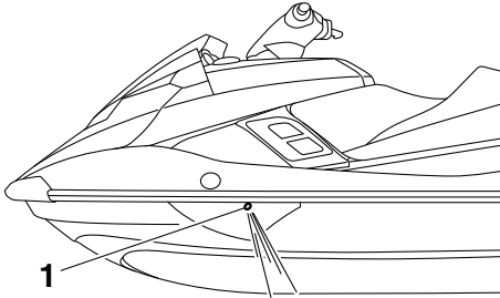
1 Kühlwasser-Kontrollauslass
